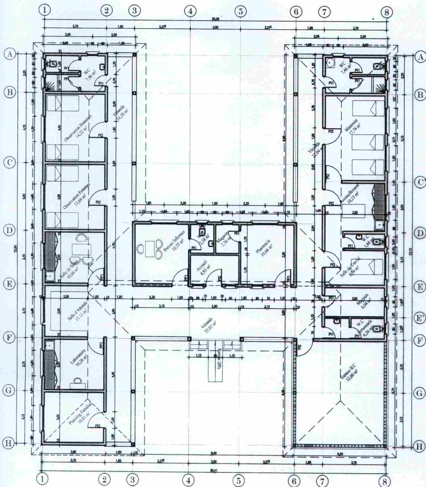
PLAN DE DISTRIBUTION
