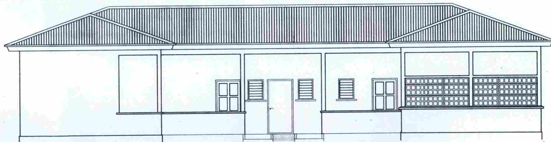
FACADE PRINCIPALE
